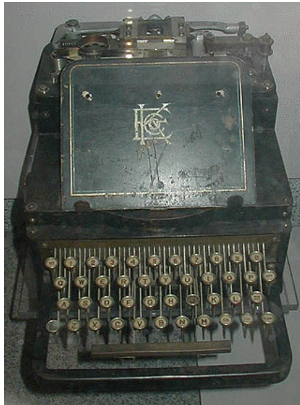
Abbildung H.9: Kleinschmidt-Perforator , gebaut um die 1920er Jahre: Mit diesem einer Schreibmaschine ähnelndem Gerät stanzt man in der kommerziellen Nachrichtenübermittlung Morsezeichen in Papier-Lochstreifen. Das Blatt mit der Text-Vorlage wurde auf der Metallplatte (in der Mitte) abgelegt. Mit dem fertigen Lochstreifen wurde der automatische Sender gesteuert, der auf diese Weise eine extrem schnelle Übertragung mit bis zu 300 Worten pro Minute erreichte. Dies waren die Vorgänger der späteren Fernschreib-Technik. [ http://www.officemuseum.com/ImagesWWW/Edward_Kleinschmidt_printing_telegraph_punched_code_on_tape_NMAH_Smithsonian_OM.jpg ]
