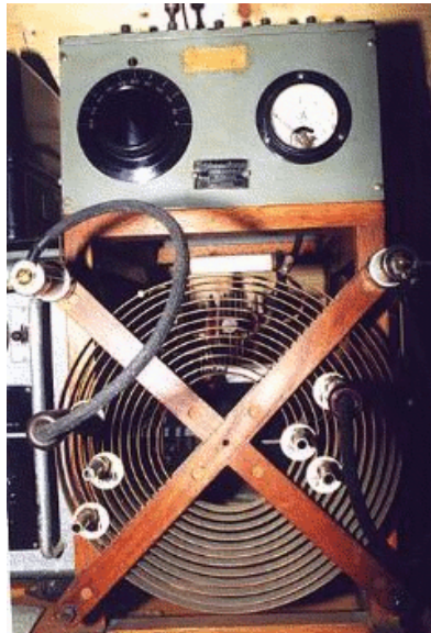
Abbildung H.11: Löschfunksender , erfunden 1906 von Max Wien. Die Funkenstrecke war auf mehrere Metallplatten mit geringem Abstand verteilt (im Gehäuse oben links). Rechts oben das Ampere-Meter für den Antennenstrom. Die Spule unten besitzt Anzapfungen für unterschiedliche Arbeitsfrequenzen. Im Gegensatz zum alten ("Knall"-)Funkensender zündet der Funke beim Durchgang durch das Schwebungsminimum nicht erneut. Dies verbessert den Wirkungsgrad und erlaubt eine Erhöhung der Funkenfrequenz bis auf 500 Hz. Deshalb wurde dieser Sender auch als Ton-Funkensender bezeichnet. [ http://www.seefunknetz.de/bilder_1/loefu250.jpg ]
